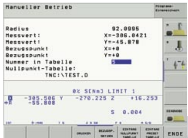
Bild 2: erweitertes Antastmenü
